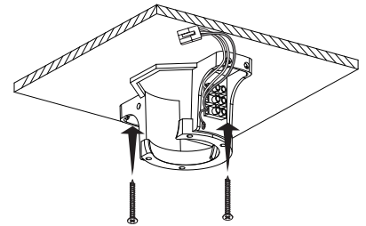
FAN ONLY MODEL
